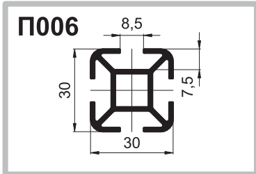
Стойка четырёхгранная
